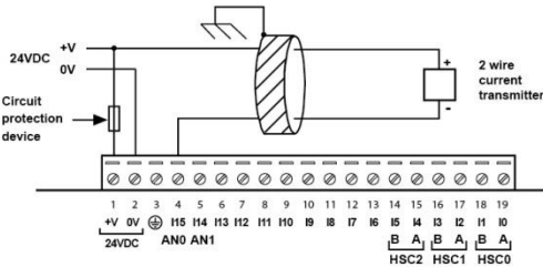
Analog input wiring, current (2 wire)
